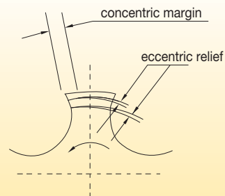
Con-Eccentric Relief
